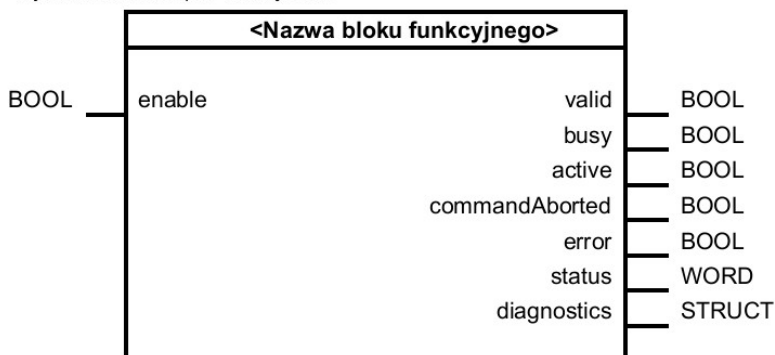
Rysunek 4-10: Reprezentacja LAD
