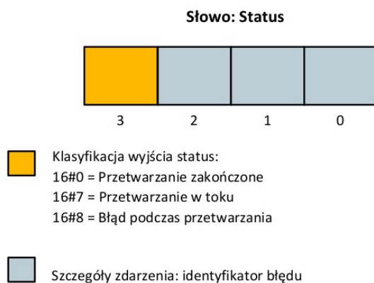
Rysunek 4-12: Struktura wyjścia "status"
