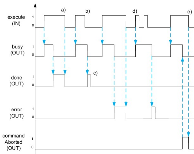
Rysunek 4-9: Diagram przejścia sygnału dla bloku funkcyjnego z parametrem wejściowym execute
