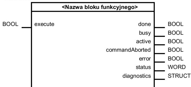
Rysunek 4-8: Reprezentacja LAD
